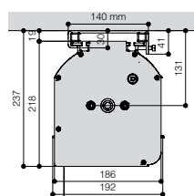
Deckenbefestigung
