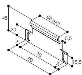
Wandhalterung
