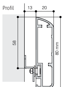
Wandhalterung
