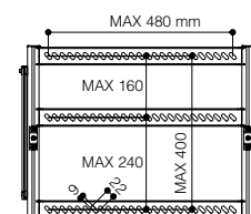
Projektor-Befestigungsplatte
