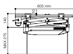
Seitenansicht eingefahren
