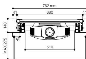
Vorderansicht eingefahren
