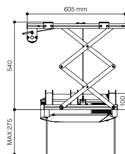
Seitenansicht ausgefahren
