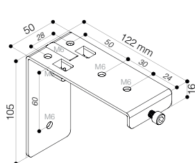
Wand-/ Deckenhalterung
